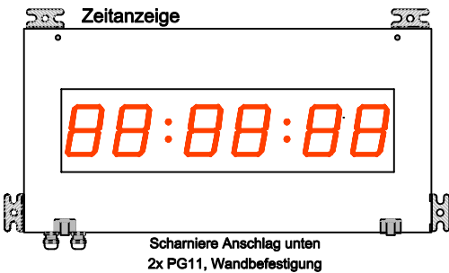
Frontansicht DA75-NU60/DxxRW
