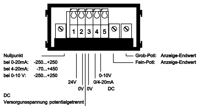
Rückansicht
