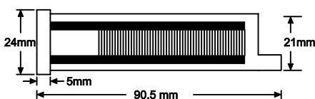
Seitenansicht
