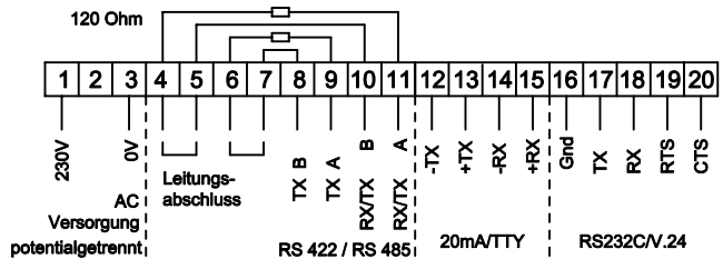
Steckbare Schraubklemmenleiste
